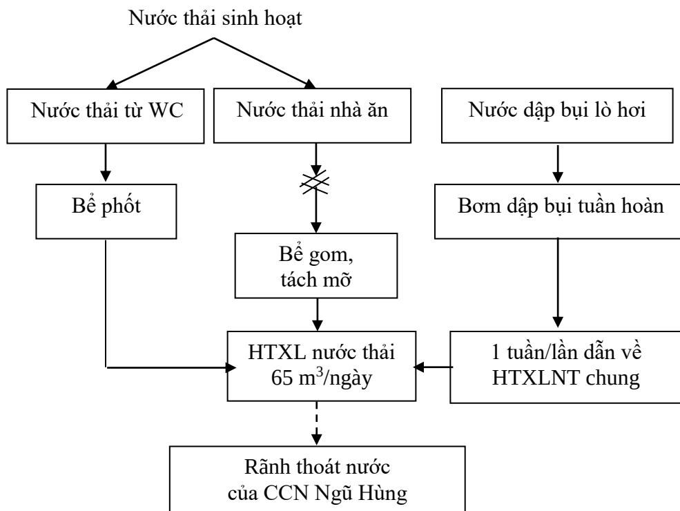
Hình 4. Sơ đồ thu gom, thoát nước thải của Nhà máy
