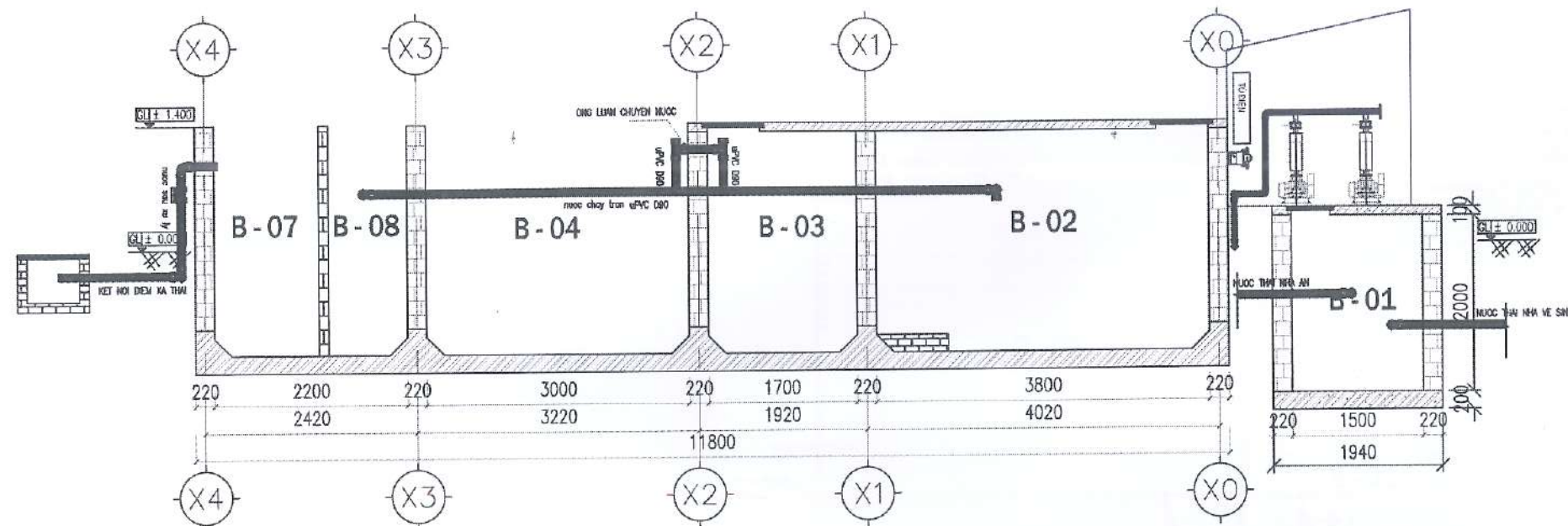
MẶT CẮT B - B
