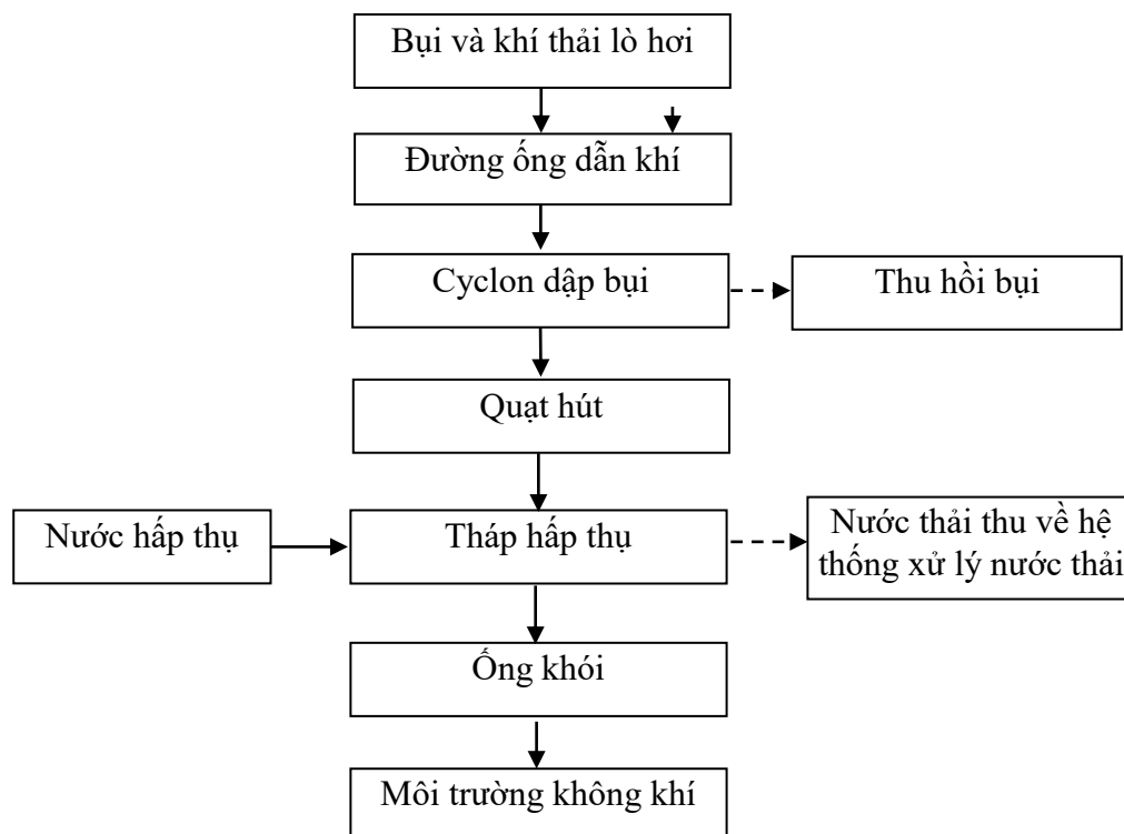
Hình 7. Sơ đồ quy trình xử lý bụi, khí thải lò hơi
