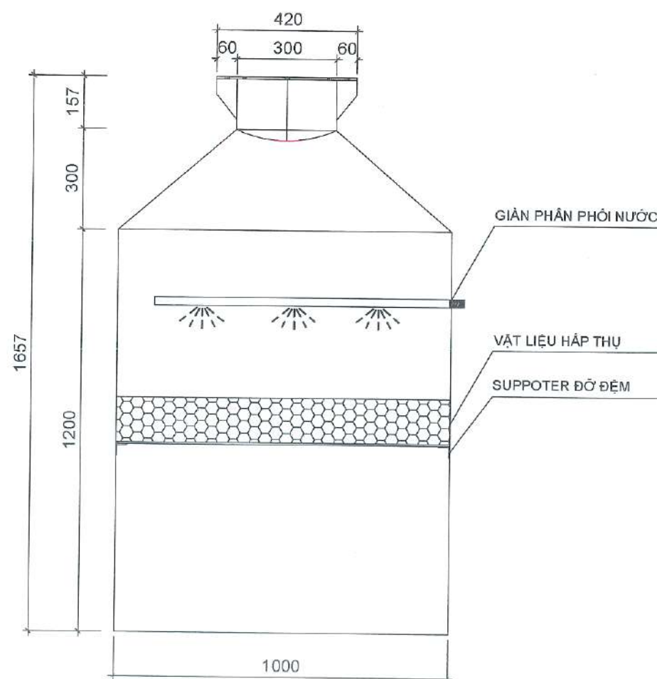
THÁP HẤP THỤ
